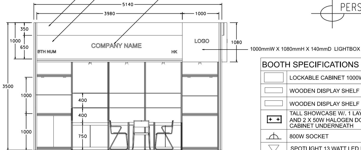
ELEVATION
